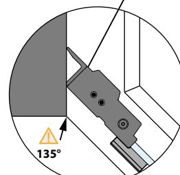
SZCZEGÓŁ B
