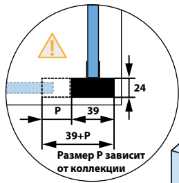
ДЕТАЛЬ А
