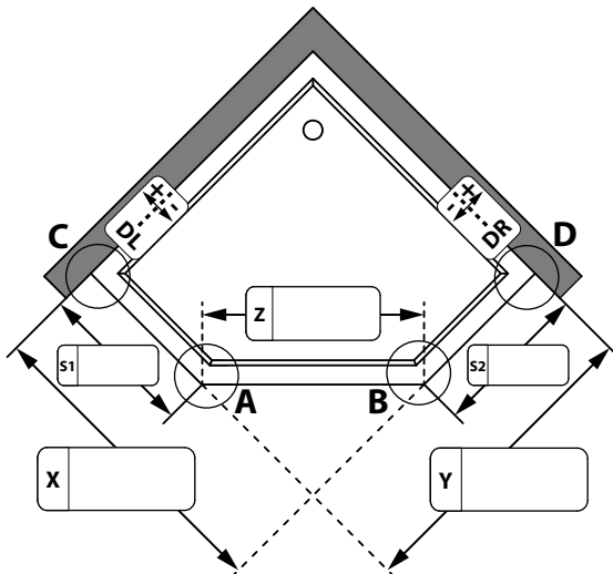
ДЕТАЛЬ E
