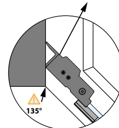
SZCZEGÓŁ B
