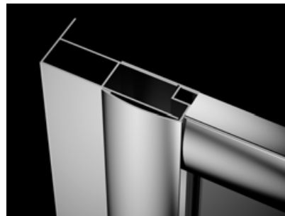
Premium Plus DWD – profil +4 cm. Standardowy profil U zastępujemy profilem poszerzającym P01-131190001.
