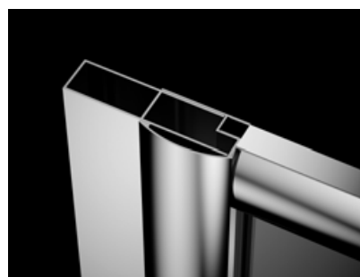
Classic – profil +4 cm. Standardowy profil U zastępujemy profilem poszerzającym Chrom - P01-124185001. Biały - P01-124185004.
