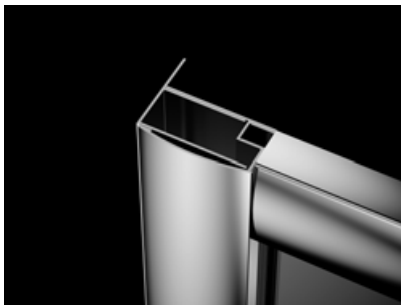
Premium Plus DWD – standardowy profil U.
