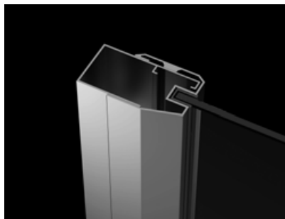
Almatea – profil +2 cm. Standardowy profil U zastępujemy profilem poszerzającym P01-110195001.
