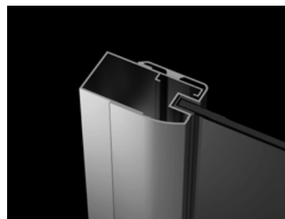
Torrenta – profil +2 cm. Standardowy profil U zastępujemy profilem poszerzającym P01-110185001.
