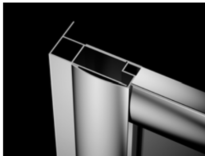
Premium Plus DWD – profil +2 cm. Standardowy profil U zastępujemy profilem poszerzającym P01-130190001.
