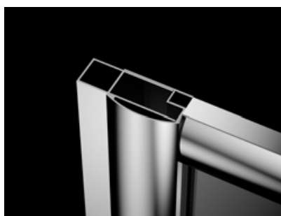
Classic – profil +2 cm. Standardowy profil U zastępujemy profilem poszerzającym Chrom - P01-112185001, Biały - P01-122185004.
