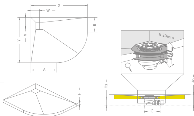
Rysunek przedstawia lewy wariant brodzika
