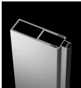
Eos, Eos II – profil +4 cm. Standardowy profil U pod magnes zastępujemy profilem poszerzającym P01-138195001.
