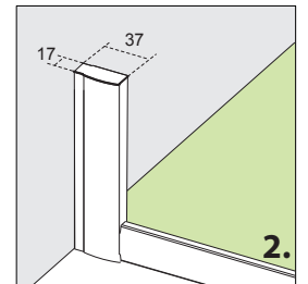
PROFIL PRZYŚCIENNY
